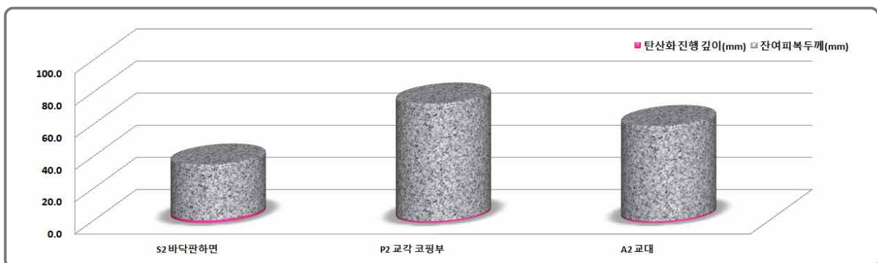
[그림 2.3.5] 탄산화깊이 및 잔여피복두께 측정결과
