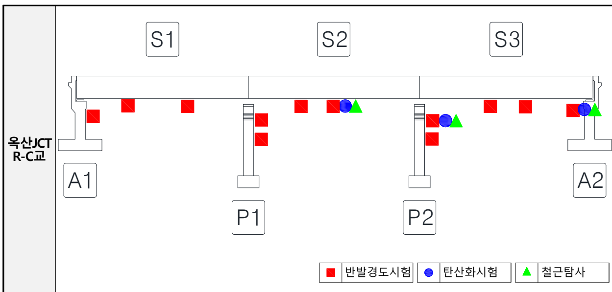
[그림 2.3.2] 비파괴시험 위치도
