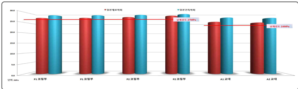
[그림 2.3.4] 반발경도법에 의한 비파괴강도 측정 결과-하부구조
