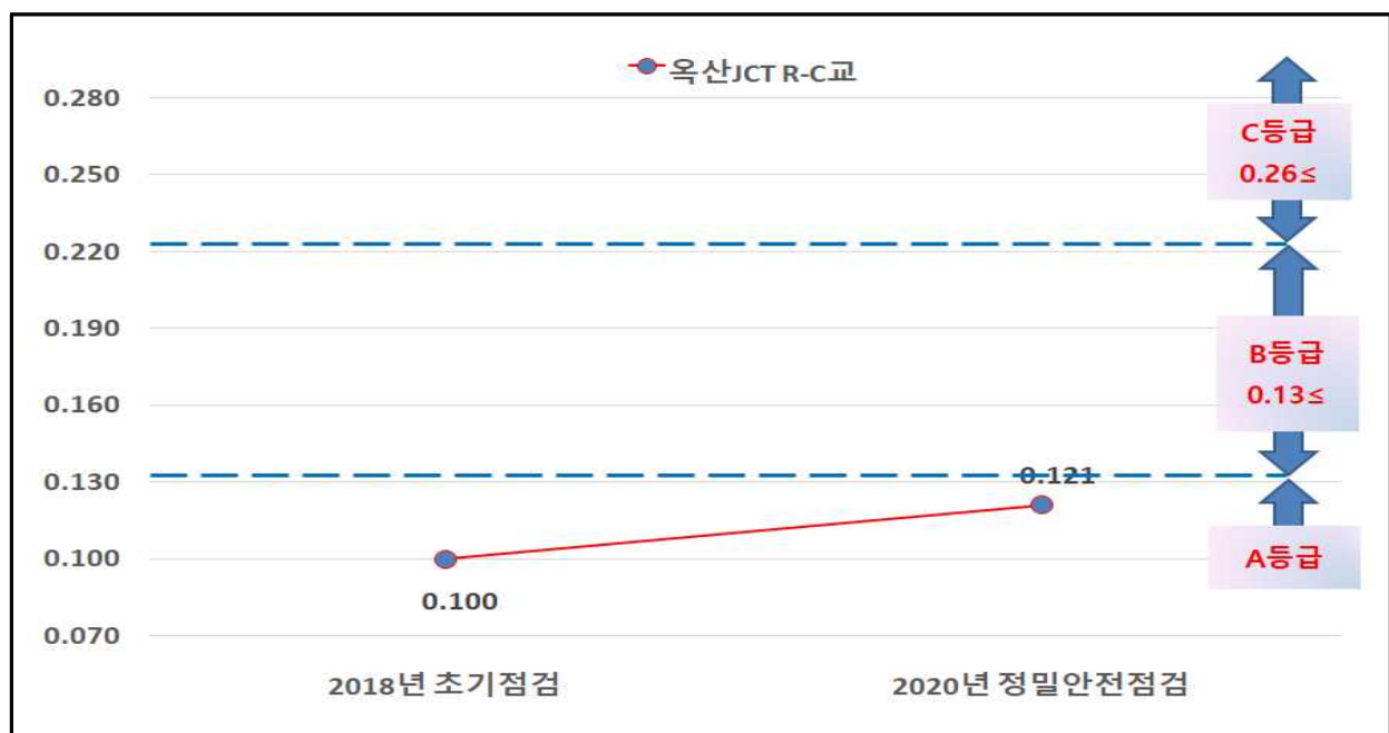
[그림 2.4.1] 옥산JCT R-C교 상태평가 결과 비교 그래프
